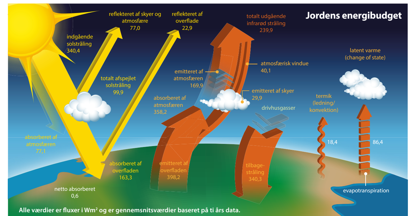
↓ Figur 3. Jordens energibudget, der viser den globale balance mellem solenergi, der når Jorden, og den energi, der forlader Jorden.
